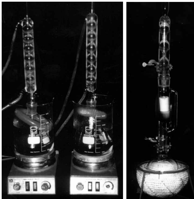
Abb. 1: Extraktionsverfahren auf dem Magnetrührer mit Wasserbad (links) und Soxhlet Extraktionsverfahren (rechts) zur Herstellung von Pflanzenextrakten.
