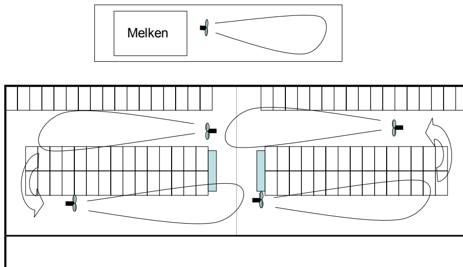
Abbildung 1: Anordnung der Umluftventilatoren im „Kreis“ zur Steigerung der Luftzirkulation (HEIDENREICH et. al. 2005)
