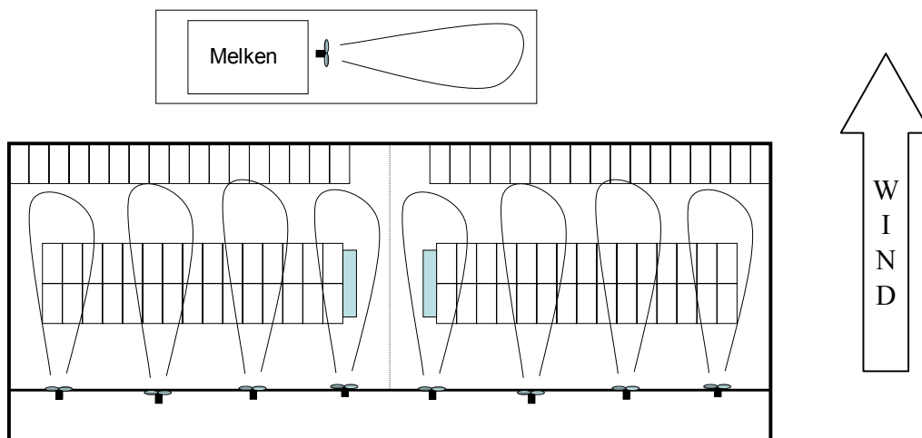
Abbildung 2: Parallelanordnung der Ventilatoren in Hauptwindrichtung zur Steigerung des Luftdurchsatzes (HEIDENREICH et. al. 2005)
