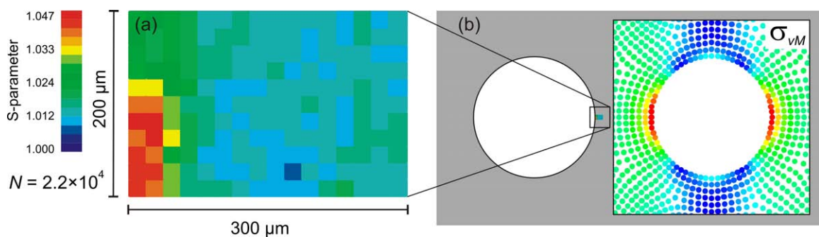
Abbildung 5.8: Teil (b) zeigt den Ausschnitt von Probengeometrie 2 um die Bohrung und die FEM Simulation der lokalen von Mises-Spannung \sigma_{vM} . Maßstabsgetreu und vergrößert (a) ist der an der BPM erfolgte Flächenscan des maximal belasteten Volumens nach 2.2 \cdot 10^4 Lastwechseln dargestellt [Eic07].
