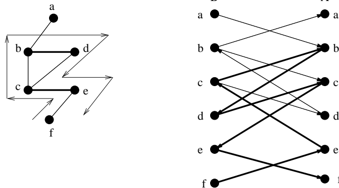
Abbildung 2.10: Besuch von [c, A] und [c, B]
