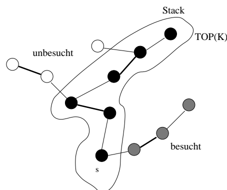
Abbildung 4.9: MDFS-Stack
