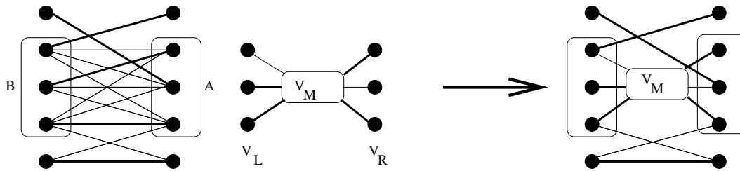
Abbildung 3.5: Korrespondierende Matchings in G und G_{C_S/C}
