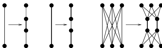
Abbildung 5.3: Ersetzung von Kanten und Cliques
