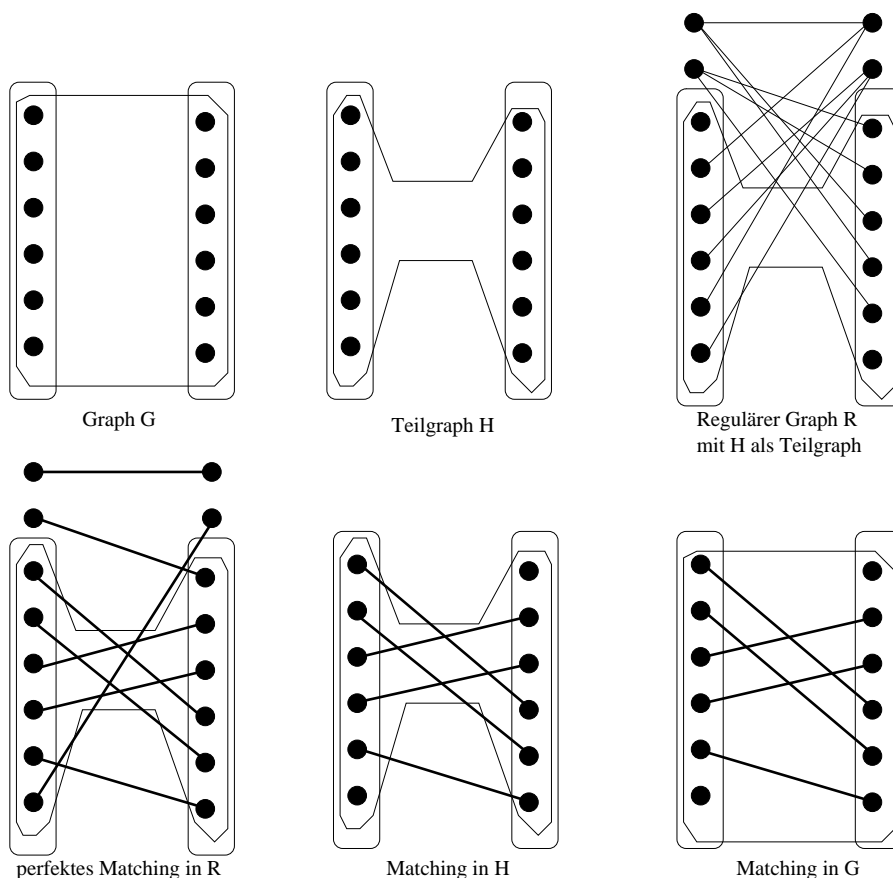
Abbildung 7.1: Veranschaulichung der Vorgehensweise
