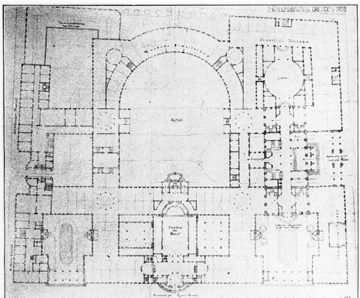
Abb. IV/37d Entwurf „Genio Loci“ von Schilling & Gräbner, Dresden, Grundriss
