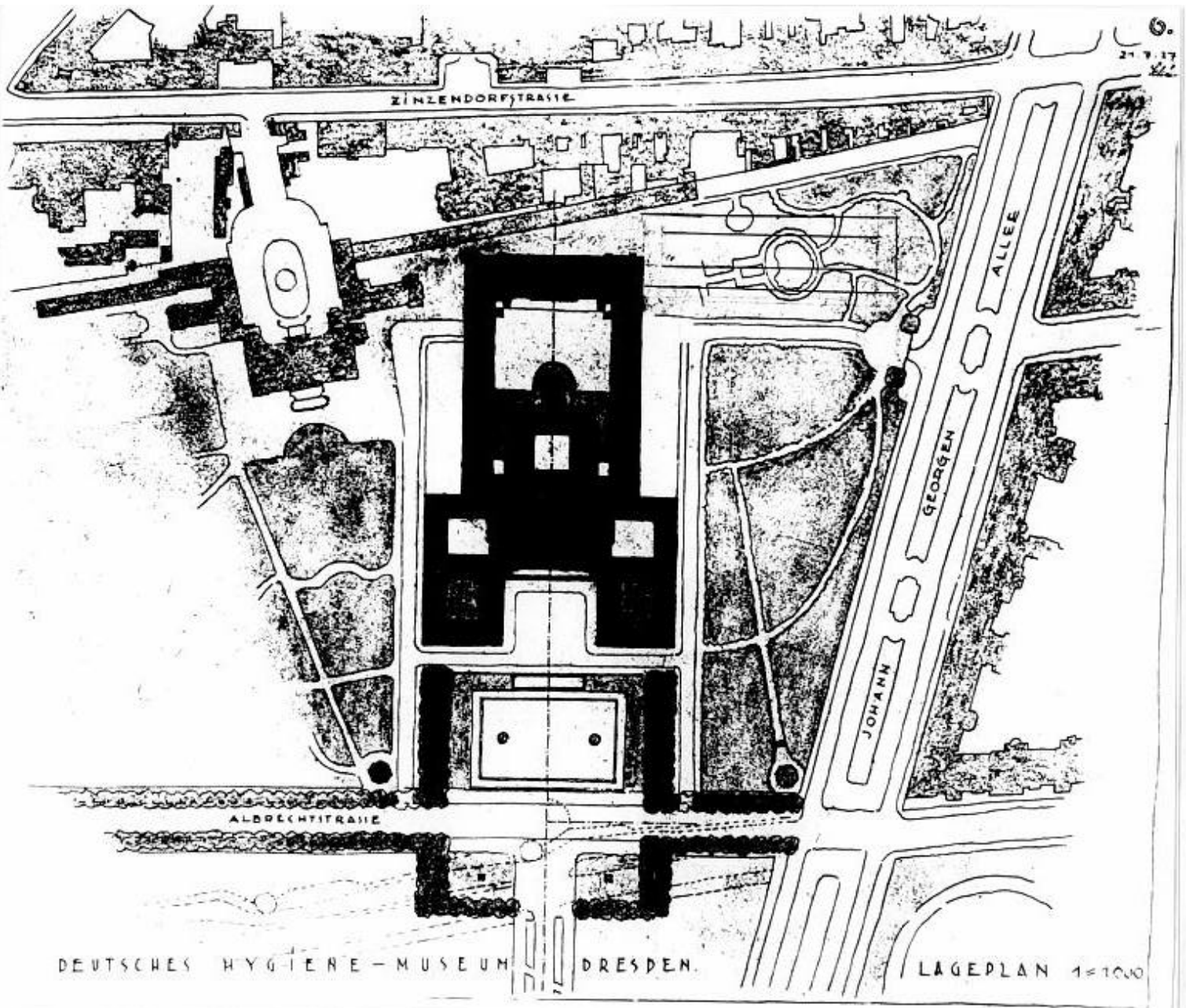
Abb. V/1 Deutsches Hygiene-Museum, Lageplan M 1:1000, datiert 21.7.27
