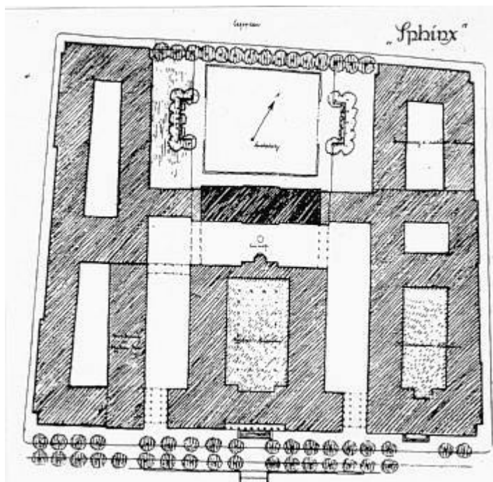
Abb. IV/48a Entwurf "Sphinx" von Zauleck & Hormann, Hamburg Lageplan
