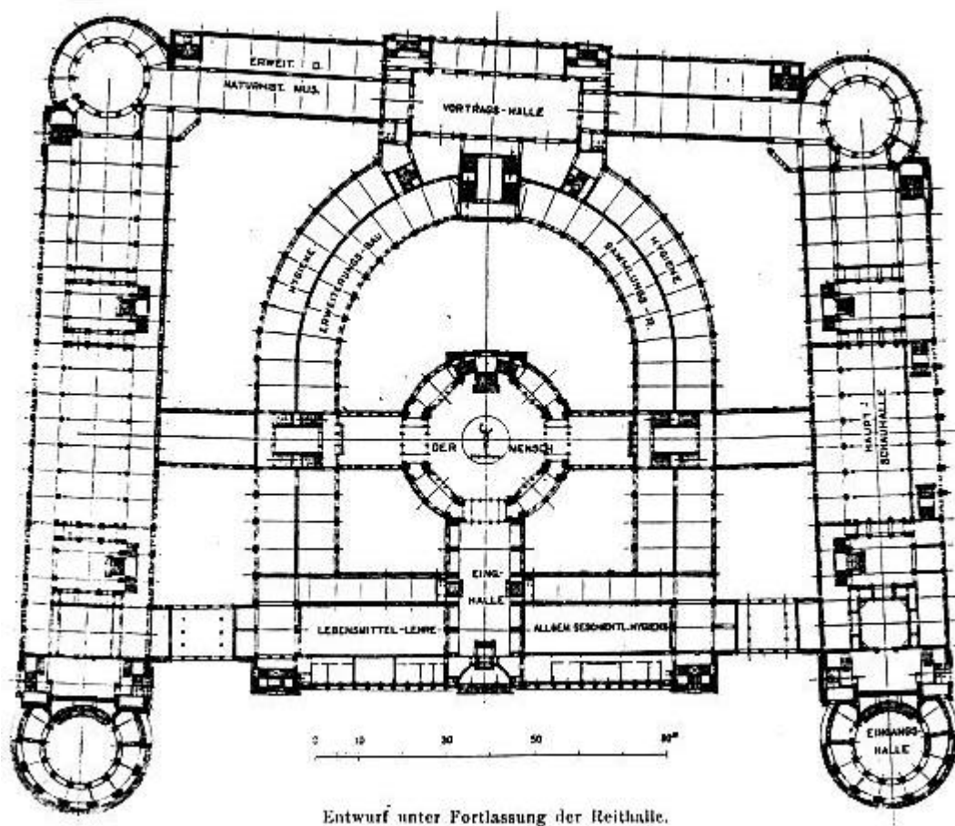
Abb. IV/28b Entwurf "Memento Viveri" von Heinrich Seeling, Berlin-Grünwald
