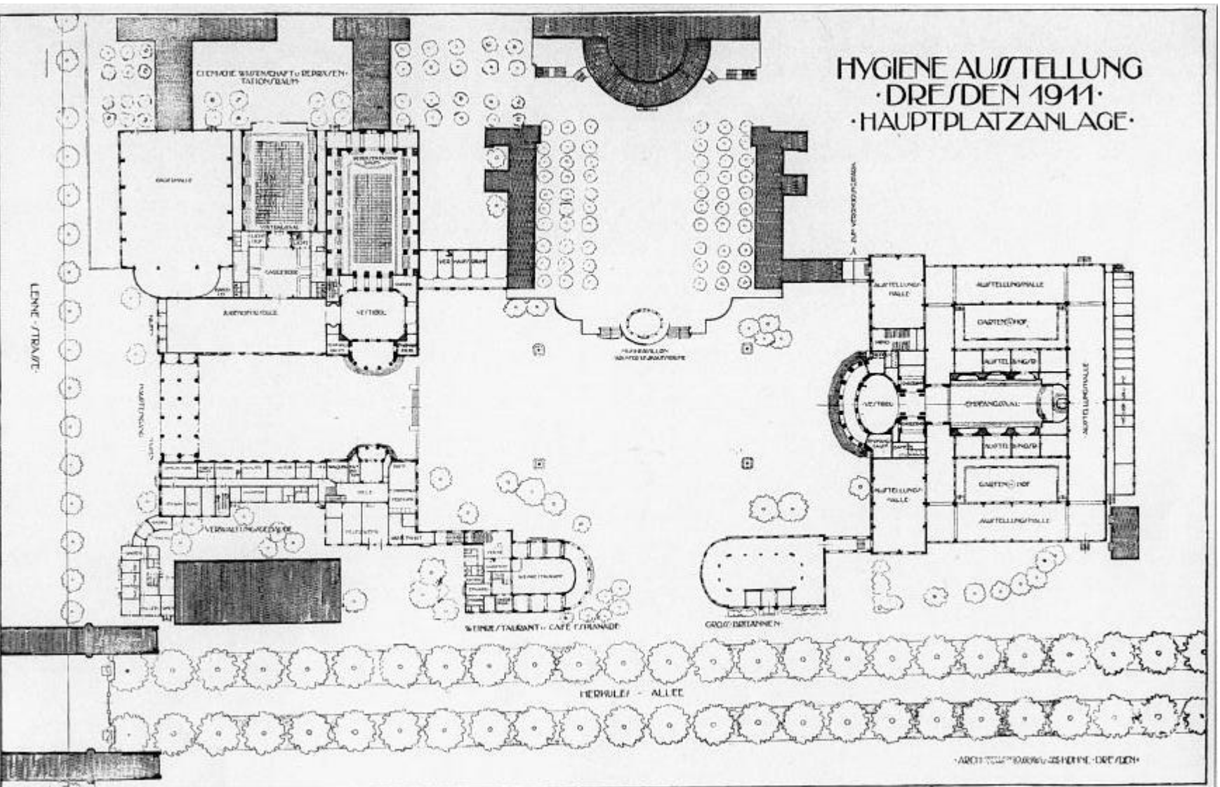
Abb. IV/7 Internationale Hygiene-Ausstellung 1911, Hauptplatzanlage Architektur Lossow & Kühne, Dresden
