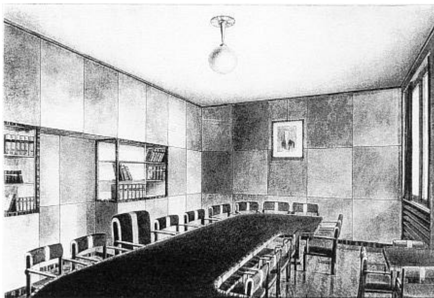
Abb. VI/34 Entwurfszeichnung Sitzungszimmer
