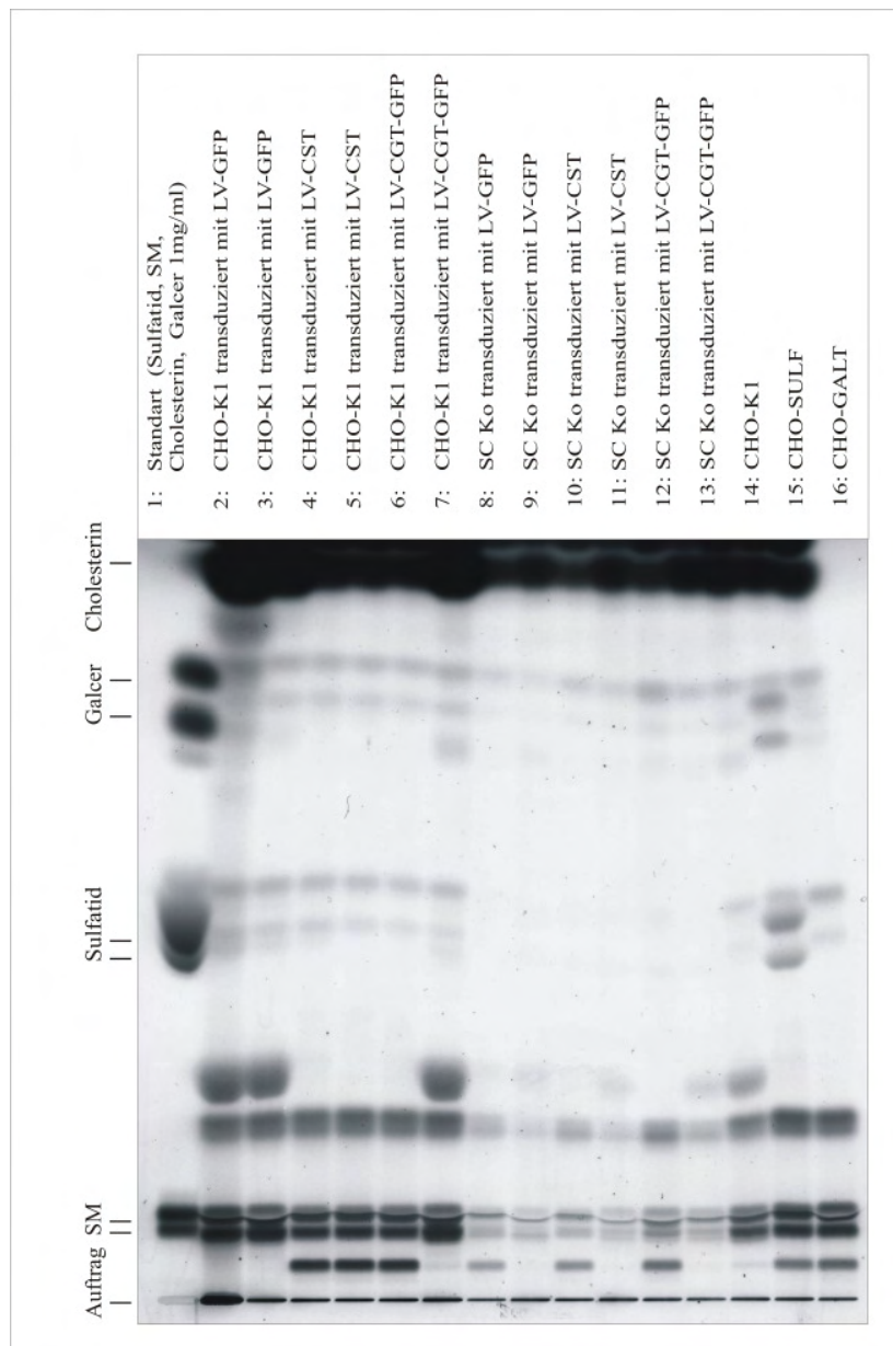
Abbildung 25: Dünnschichtchromatographie von Lipiden aus transduzierten, ASA-defizienten Schwann-Zellen und transduzierten CHO-K1-Zellen
