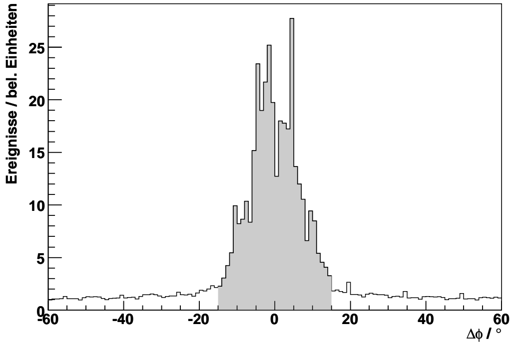
Abbildung 7.5: \phi -Winkeldifferenz \Delta\phi zwischen allen Teilchen, die im CB registriert wurden, und den getroffenen PID-Streifen. Lag die Differenz zu einem Streifen innerhalb des Fensters von \pm 15^\circ , so wurde das Teilchen als geladen gewertet.
