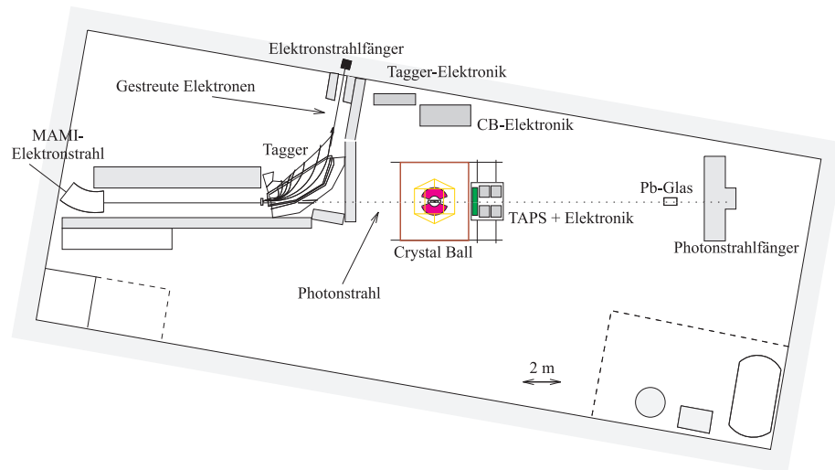
Abbildung 3.4: Grundriss der A2-Experimentierhalle
