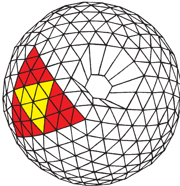
Abbildung 3.10: Geometrie des Crystal Ball. Zu erkennen ist ein Bereich, der für den Strahleneintritt freigelassen wurde. Dieser hatte eine hexagonale Form. Farblich markiert ist eine Seite des Ikosaeders („Major Triangle“). Diese ist unterteilt in vier kleine Dreiecke („Minor Triangle“). Jedes dieser Dreiecke besteht aus neun Kristallen.
