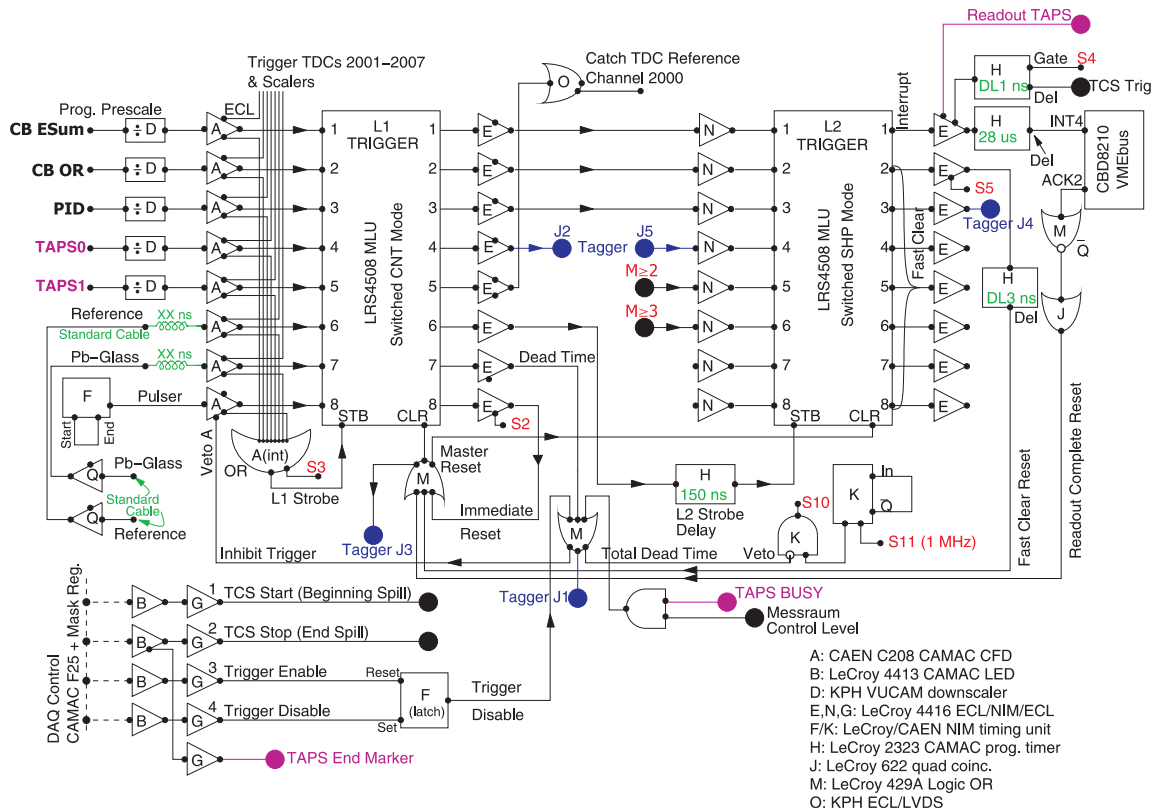
Abbildung 4.11: Schaltung der Trigger-Register zur Auswertung der Energiesummen- und Multiplizitätsinformationen. Der Level-1-Trigger wurde durch die Energiesumme im CB gebildet; im Level-2 wurde die Bereichsmultiplizität von CB und TAPS ausgewertet.
