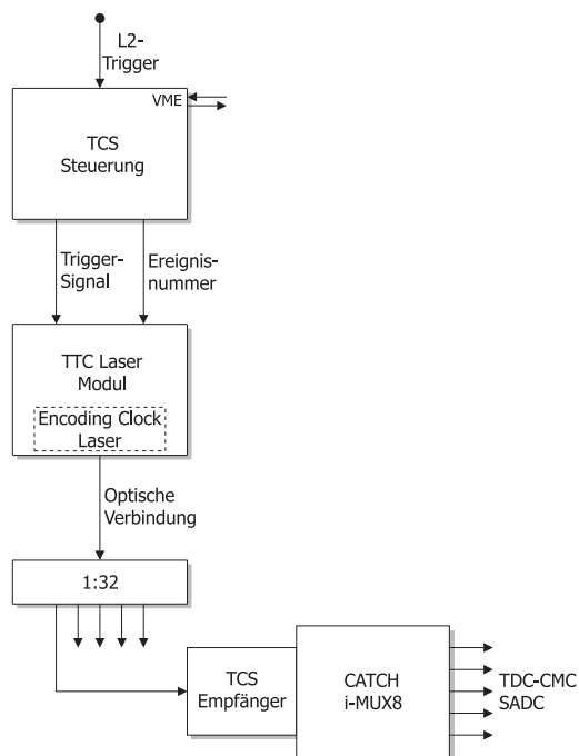
Abbildung 4.12: Schema des Trigger-Kontrollsystem (TCS). Es diente der Verteilung von Trigger-Informationen an die CB-Ausleseelektronik.
