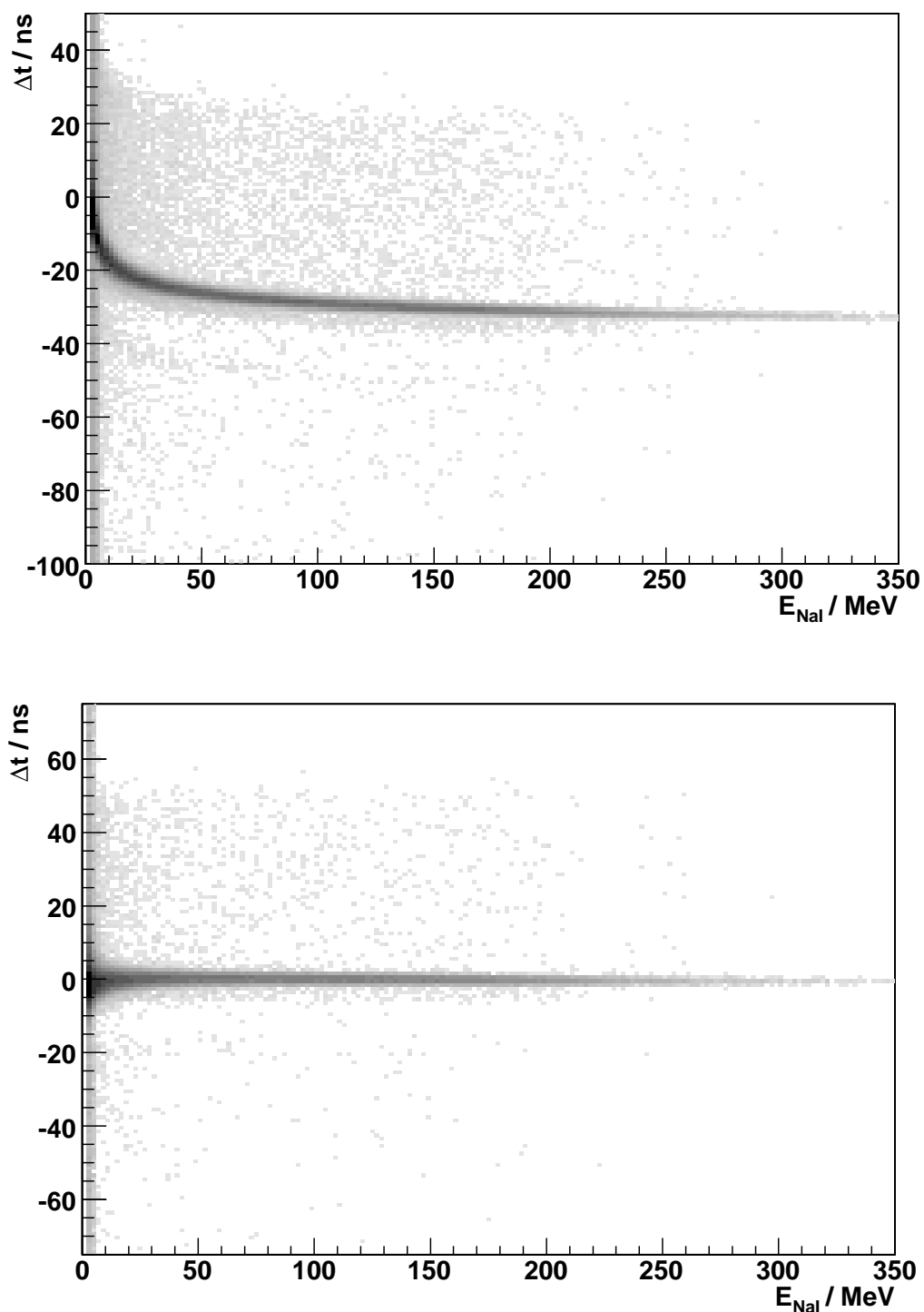
Abbildung 7.4: Pulshöhenabhängigkeit der Zeitinformation eines einzelnen CB-Kristalls. Auf den y-Achsen ist die Zeitdifferenz zum vom Proton getroffenen PID-Szintillator aufgetragen, auf der x-Achse die Energie der entsprechenden NaI-Kanäle. Oben: Vor der Walk Correction . Unten: Nach dem Zeitabgleich.
