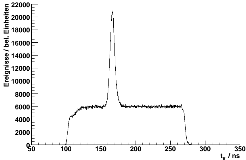
Abbildung 3.9: Tagger-Zeitspektrum. Deutlich zu erkennen ist der Pik (FWHM = 9,7 ns) von Ereignis-Elektron-Paaren, der aus dem Untergrund herausragt.
