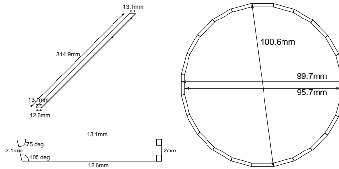
Abbildung 3.14: Der Particle-Identification-Detektor. Links ist die Form eines Szintillatorstreifens zu sehen. Rechts ist ein Querschnitt des PID gezeigt.
