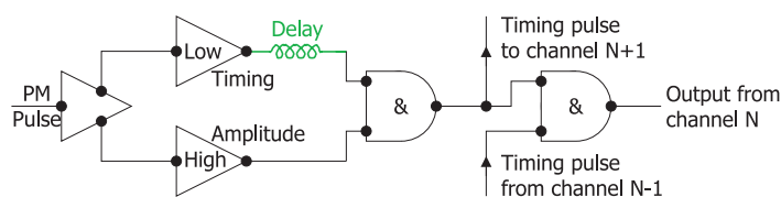
Abbildung 4.1: Tagger-Auslesekarten. Zwei benachbarte Szintillatoren wurden in Koinzidenz geschaltet und bildeten dadurch einen Tagger-Kanal.
