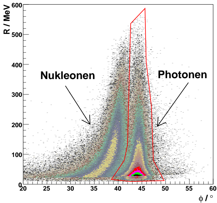
Abbildung 7.11: Pulsformanalyse der \text{BaF}_2 -Signale. Oben: Aufgetragen ist die Energiedeposition im kurzen gegenüber der im langen Integrationsfenster. Unten: Darstellung in den Koordinaten R und \phi nach Gleichung 7.19. Zu sehen sind der Photonennast bei ca. 45^\circ und links davon die Nukleonen. Der markierte Bereich zeigt den Schnitt auf Photonen zur Teilchenidentifizierung.
