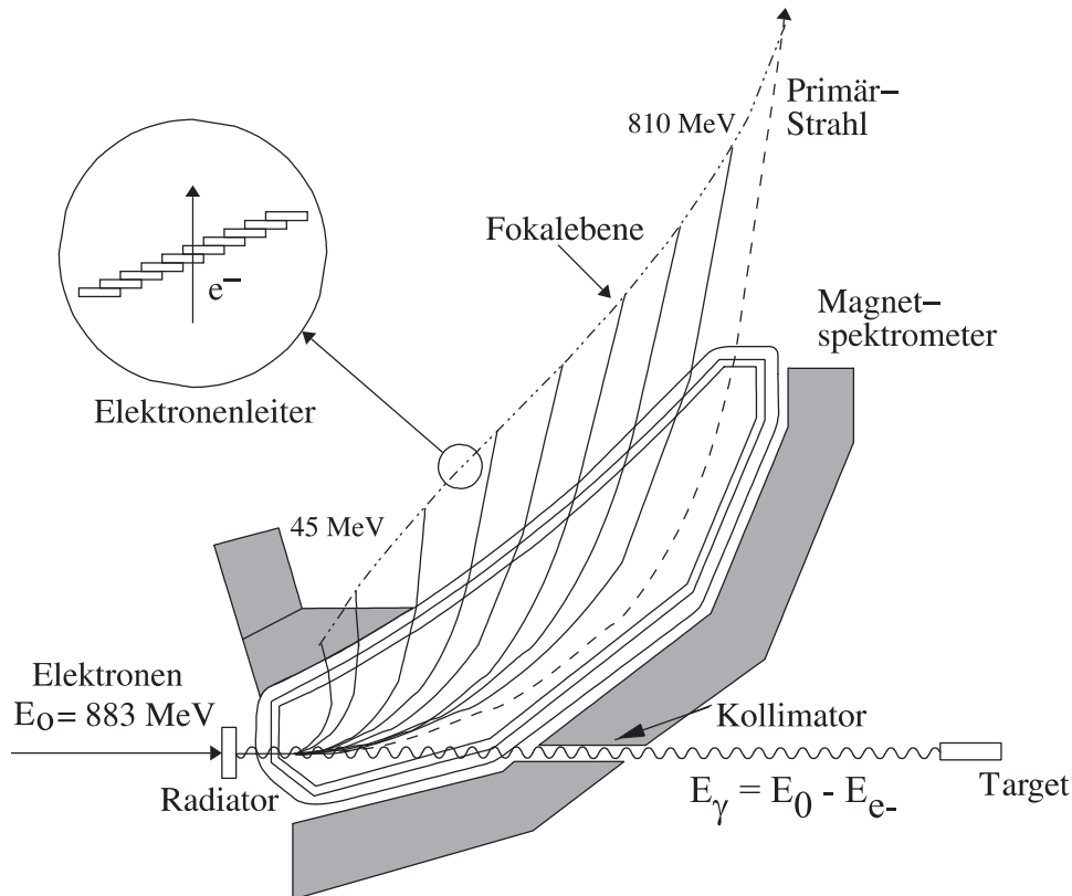
Abbildung 3.5: Der Glasgow-Mainz-Tagger
