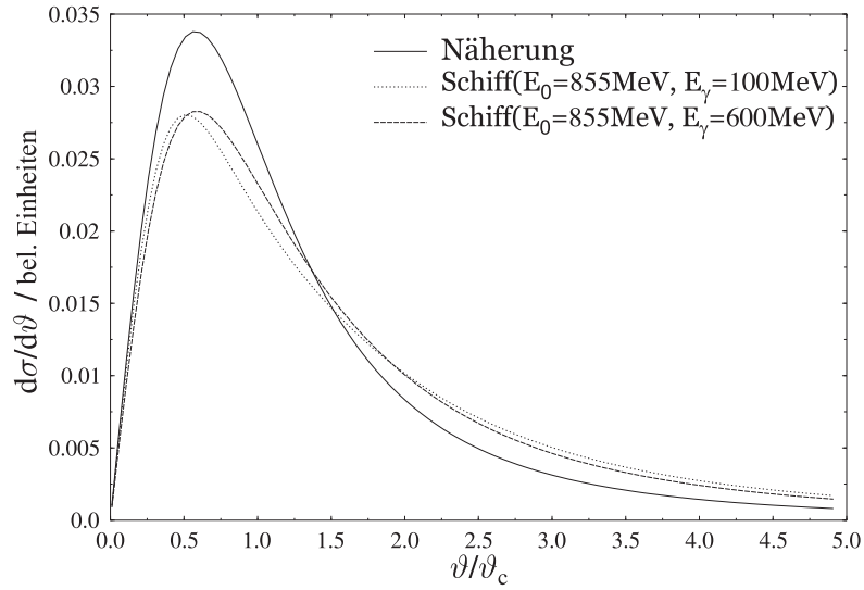
Abbildung 3.8: \vartheta -Winkelverteilung der Bremsstrahlungsphotonen. Gezeigt werden die in Gleichung 3.3 gegebene Näherung und realistischere Rechnungen (Schiff).
