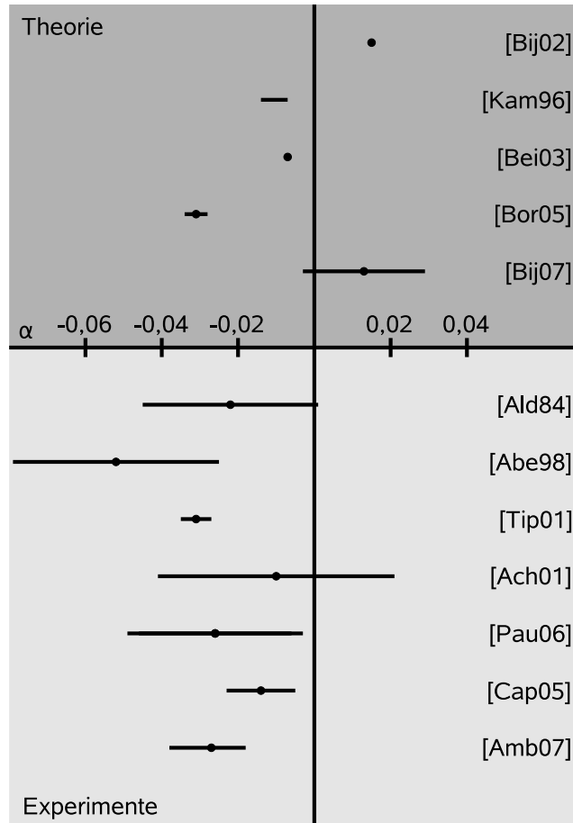
Abbildung 1.1: Vergleich einiger bisher veröffentlichter Werte für den Dalitz-Plot-Parameter \alpha aus der Theorie und den Experimenten. Die erste Messung ([Bag70]) wurde ausgelassen, da sie auf Grund ihrer geringen Statistik keine Relevanz besitzt.
