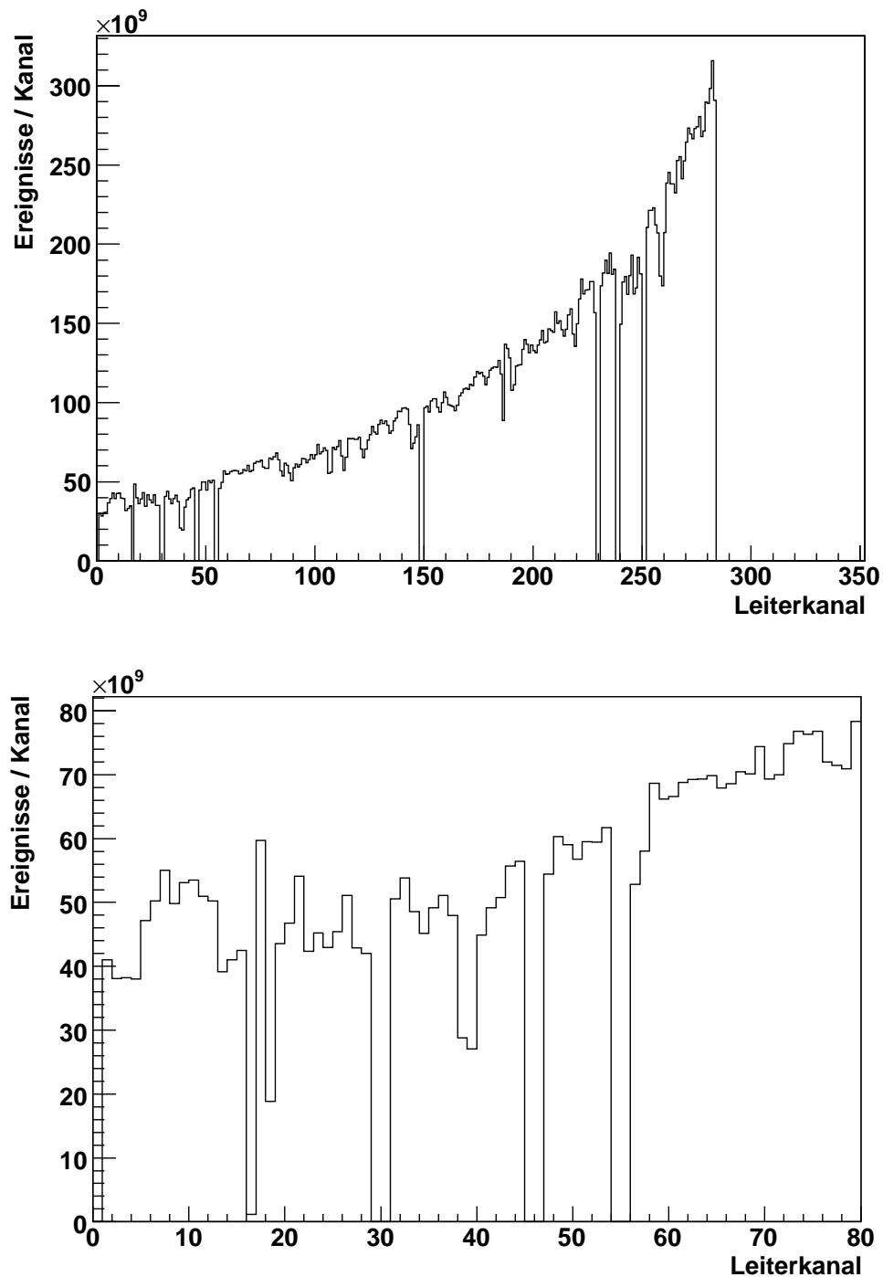
Abbildung 3.7: Bremsstrahlungsspektrum der Tagger-Leiter. Oben: Zu erkennen ist der 1/E_\gamma Verlauf. Unten: In den \eta -Experimenten sind die Kanäle 0 ( E_\gamma \approx 819 MeV) bis 79 ( E_\gamma \approx 682 MeV) verwendet worden, um sich auf den Bereich der \eta -Produktion (Schwelle: ca. 707 MeV) zu beschränken. Durch Ineffizienzen in den einzelnen Tagger-Kanälen ist die durch die Energiebreiten verursachte Überhöhung hier nur undeutlich zu erkennen.
