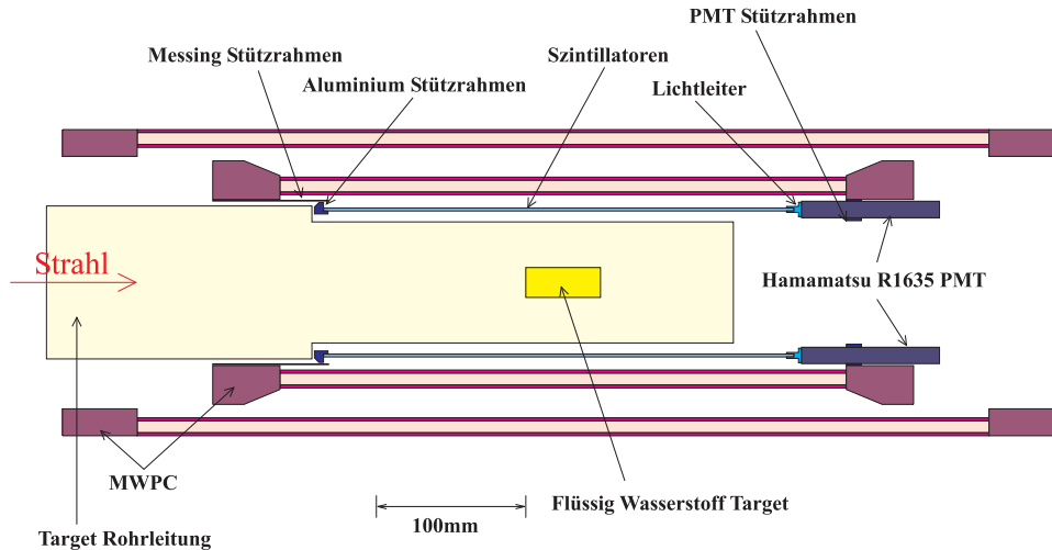
Abbildung 3.2: PID innerhalb der MWPC (Multi Wire Proportional Chamber = Vieldraht-Proportionalkammer); im Zentrum ist das Flüssigwasserstoff-Target zu sehen.
