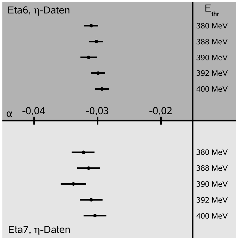
Abbildung 9.11: Ergebnisse der Testreihen zum Schnitt auf die CB-Energiesumme im Trigger, gegliedert nach den Hauptanalysen. Die Trigger-Energieschwelle hatte keinen Einfluss auf die MDM-Daten. Deshalb wurde dieser Test nur auf die \eta -Daten angewandt. Von oben nach unten sind die \alpha jeweils für einen Schnitt von E_{thr} = 380 MeV, E_{thr} = 388 MeV, E_{thr} = 390 MeV, E_{thr} = 392 MeV und E_{thr} = 400 MeV eingezeichnet.
