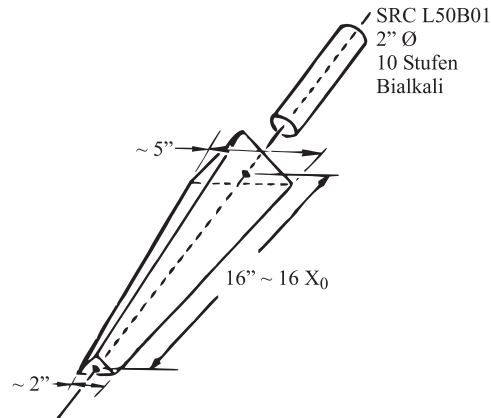
Abbildung 3.13: Ein einzelnes NaI-Modul. Insgesamt gab es im CB 11 verschiedene Kristallmodule mit leicht unterschiedlichen Abmessungen.
