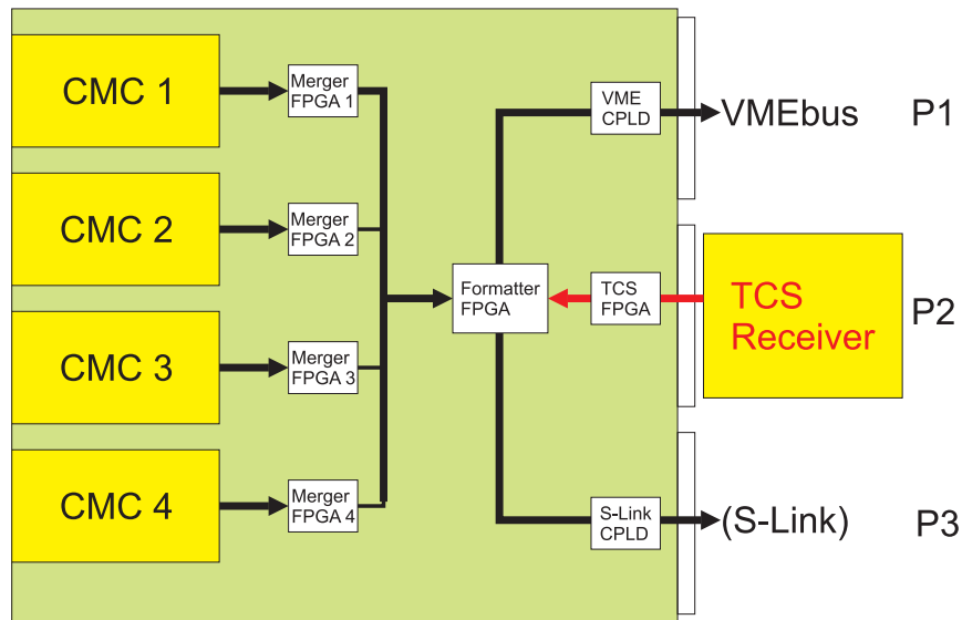
Abbildung 4.5: Schematischer Aufbau des CATCH-Moduls
