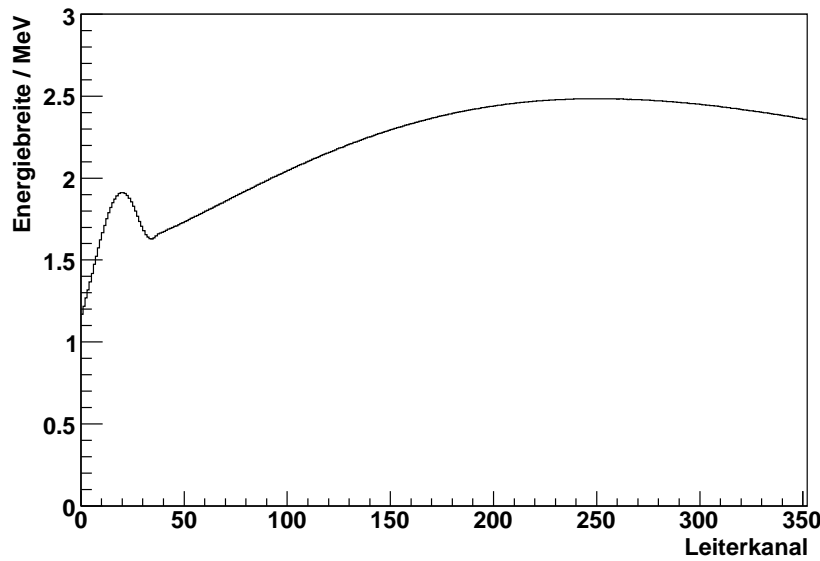
Abbildung 3.6: Energiebreiten der einzelnen Tagger-Kanäle. Zu niedrigen Kanälen zeigt sich eine deutliche Überhöhung der Breiten. Sie entsteht durch die schlechtere Fokussierung des Dipolspektrometers in diesem Bereich [Hal96].
