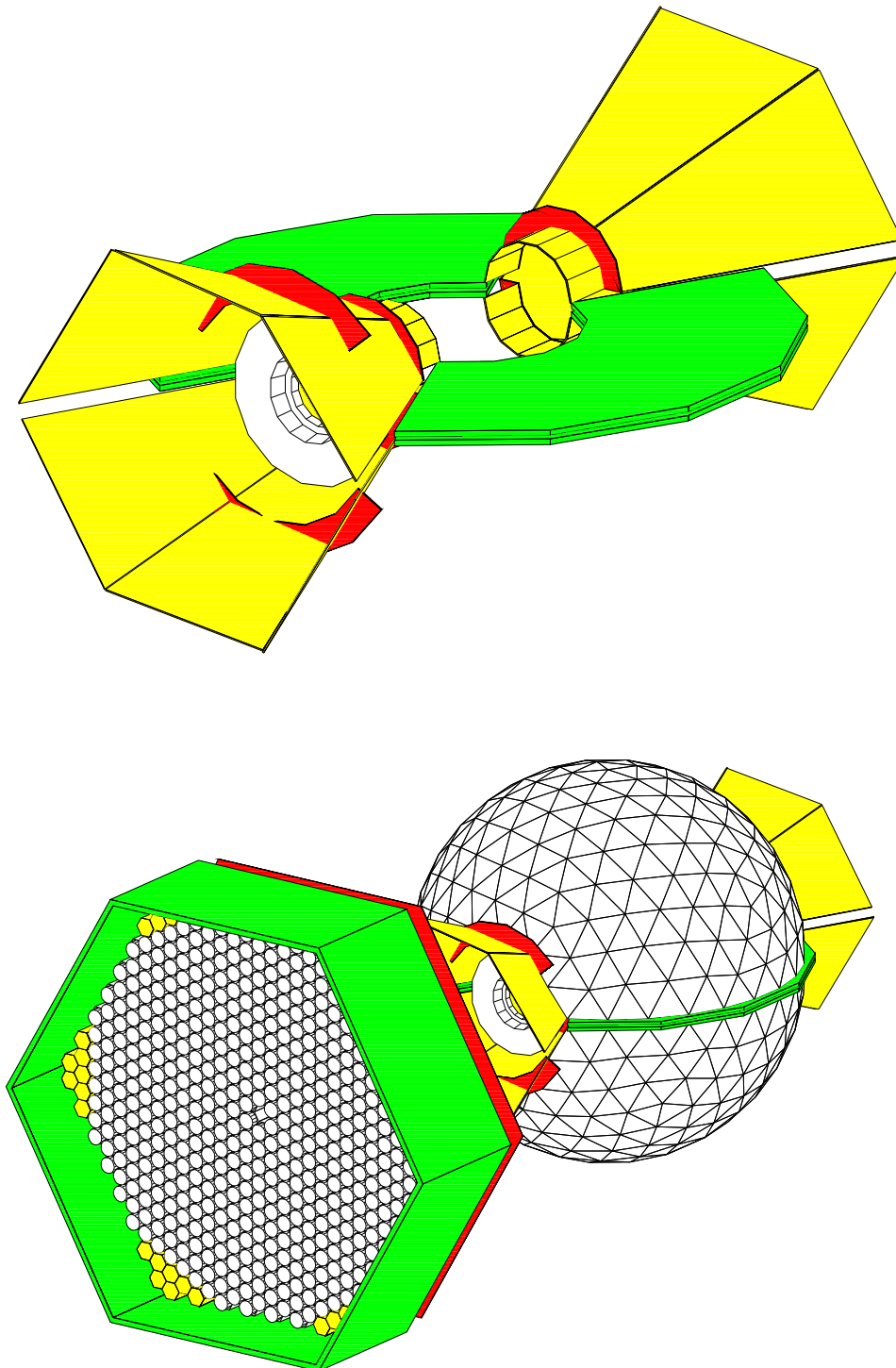
Abbildung 5.4: Detektorgeometrie in der Simulation. Oben : Crystal Ball-Stahlstrukturen. Unten : Die gesamte Detektoranordnung, wie sie in der Simulation verwendet wurde. Der Strahl kommt jeweils von rechts. Im Strahlaustrittsbereich sind auch die Volumen, die die Kabel und Elektronik des PID und der Drahtkammern repräsentierten, zu sehen.
