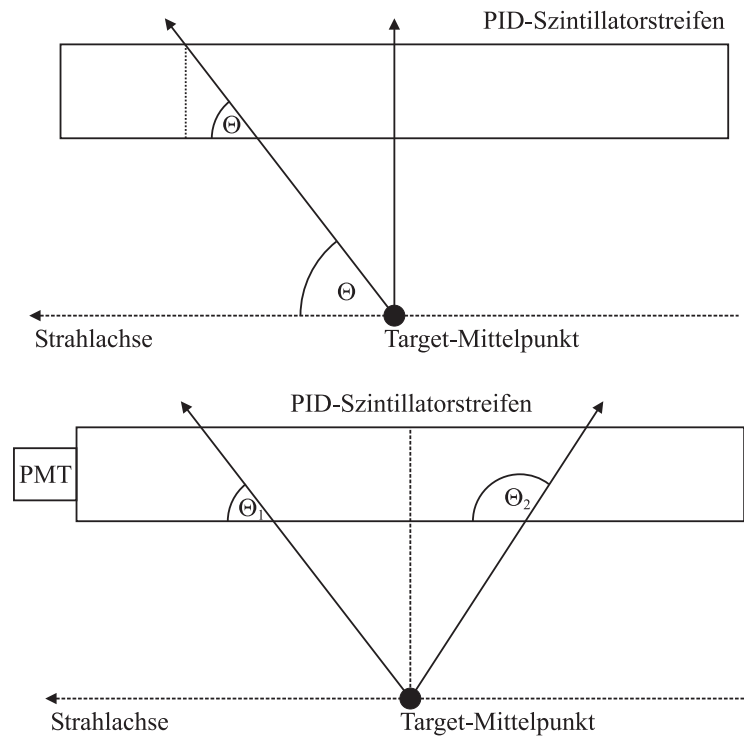
Abbildung 7.6: Korrekturen der PID-Energien. Oben: Teilchen, die nicht unter einem Winkel von \theta = 90^\circ durch den Szintillator geflogen sind, verloren auf Grund der längeren Wegstrecke mehr Energie. Sie wurden auf die Teilchenbahn mit einem Winkel von 90^\circ normiert. Unten: Für das Szintillationslicht von Teilchen mit großen \theta -Winkeln war die Strecke zum Photomultiplier länger. Deshalb kam es hier zu größeren Lichtverlusten. Dieser Unterschied wurde durch Korrekturfaktoren ausgeglichen.
