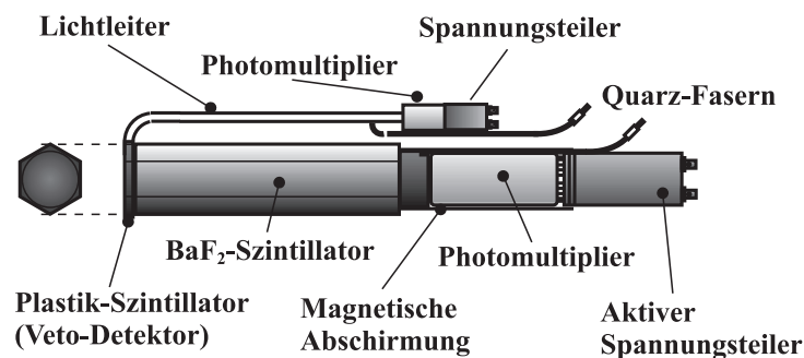
Abbildung 3.16: Einzelnes \text{BaF}_2 -Modul mit Photomultiplier und Veto-Detektor
