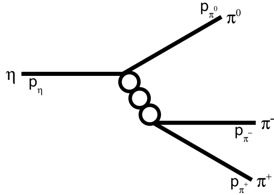
Abbildung 2.5: Rückstreuereffekte in der theoretischen Berechnung nach [Bor05]. Gezeigt ist ein möglicher Beitrag der Endzustandswechselwirkungen für den Kanal \eta \rightarrow \pi^+ \pi^- \pi^0 .
