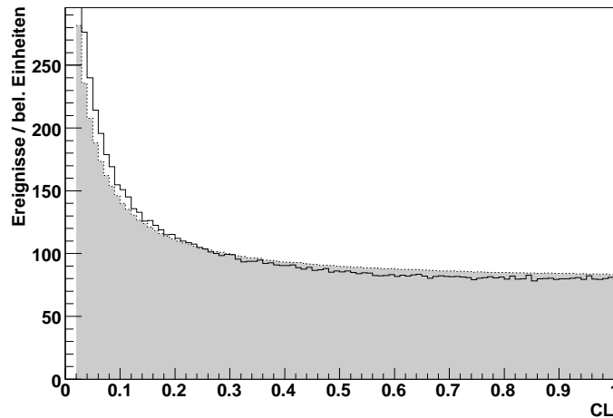
Abbildung 8.5: Confidence Level der zweiten kinematischen Anpassung. Grau hinterlegt ist die Simulation zu sehen, in schwarz das Resultat der gemessenen Daten. Die Gleichverteilung bei höheren Werten spiegelt wahre Ereignisse der Reaktion \gamma p \rightarrow \eta p \rightarrow 3\pi^0 p wieder.
