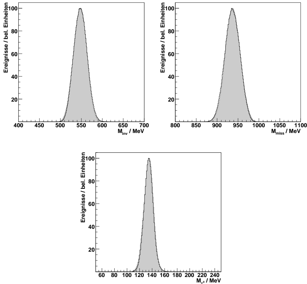
Abbildung 8.7: Massenverteilungen der unveränderten Photonenvierimpulse nach der Selektion durch die zweite kinematische Anpassung. Oben links : Invariante Masse aller sechs Photonen. Die Pikposition wurde zu M_{\text{inv}} = 547,5 MeV bestimmt. Oben rechts : Fehlende Masse aller sechs Photonen. Die Pikposition wurde zu M_{\text{miss}} = 936,9 MeV bestimmt. Unten : Invariante Masse der drei als Pionen bestimmten Photonenaare. Die Pikposition wurde zu M_{\pi^0} = 134,4 MeV bestimmt.
