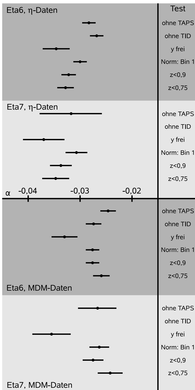
Abbildung 9.12: Ergebnisse weiterer Testreihen, gegliedert nach den vier Standardanalysen. Die Untersuchung der systematischen Unsicherheit der Teilchenidentifikation (ohne TID) konnte nur für die Eta6-Analysen angewendet werden.
