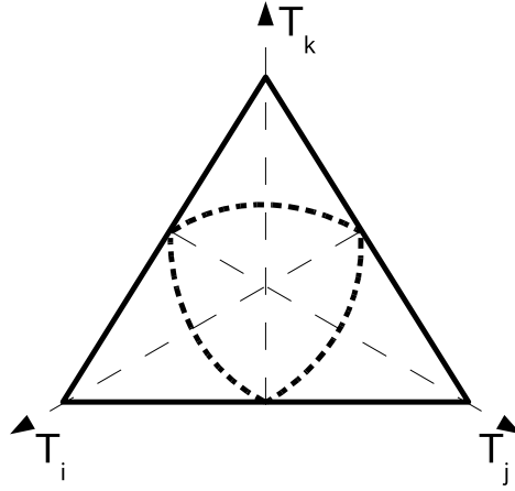
Abbildung 2.6: Schematische Darstellung des Dalitz-Diagramms. Die drei Achsen stehen für die kinetischen Energien der Pionen aus dem Zerfall \eta \rightarrow 3\pi . Durch die Energieerhaltung werden die Energien auf Kombinationen innerhalb des Dreiecks beschränkt. Die zusätzlich geltende Impulserhaltung läßt nur noch Punkte innerhalb der runden inneren Grenzen (gestrichelt) zu.
