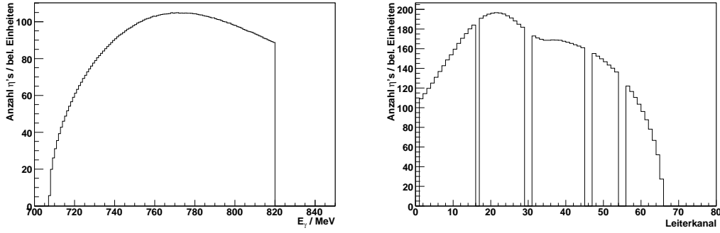
Abbildung 5.2: Energieverteilung der simulierten Strahlphotonen. Links : Energieverteilung der Photonen aufgebaut aus den erzeugten Kinematiken. Rechts : Energieverteilung der Photonen umgerechnet auf die verwendeten Tagger-Kanäle. Die Überhöhung bei kleinen Kanalnummern resultierte aus den wahren Energiebreiten der einzelnen Tagger-Kanäle (siehe Abbildung 3.6). Die Lücken in diesem Spektrum entsprechen beschädigten Kanälen, die in der Simulation nicht ausgewertet wurden.
